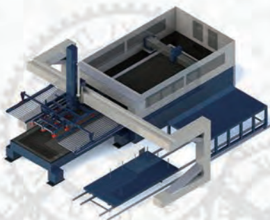
激光上下料机器人（ALG）
