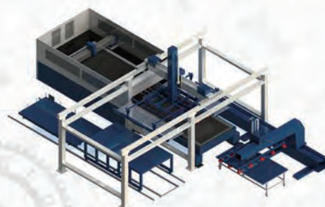
激光上下料机器人（ALG）
