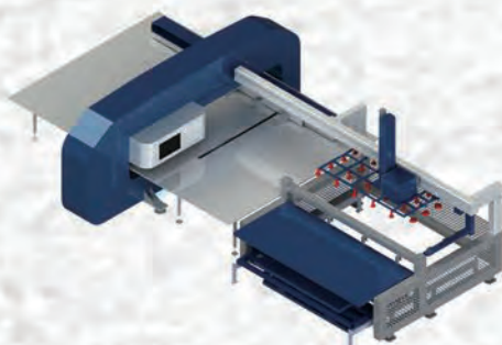
APF冲床上下料
